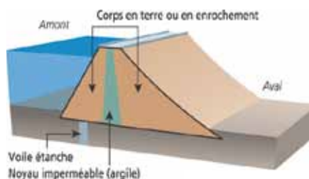
Barrage poids en terre ou en enrochement
