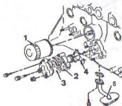
Fig. 28-b- : Vue éclatée du circuit de graissage.
