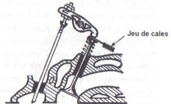
Fig. 26 : Réglage des soupapes.
